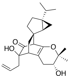
spirooliganone C
